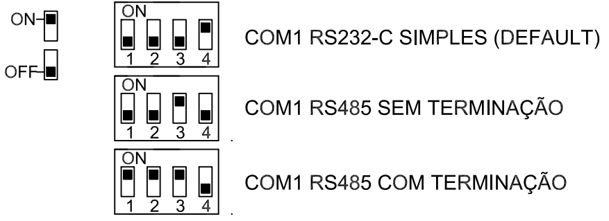
PLACA DE COMUNICAÇÃO DIP 4 (RS232-C/RS485)
