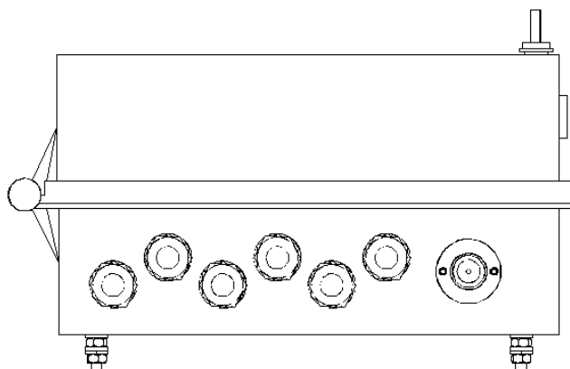
Figura 3 - ACOS225 BM LT, vista inferior, entrada para cabos
