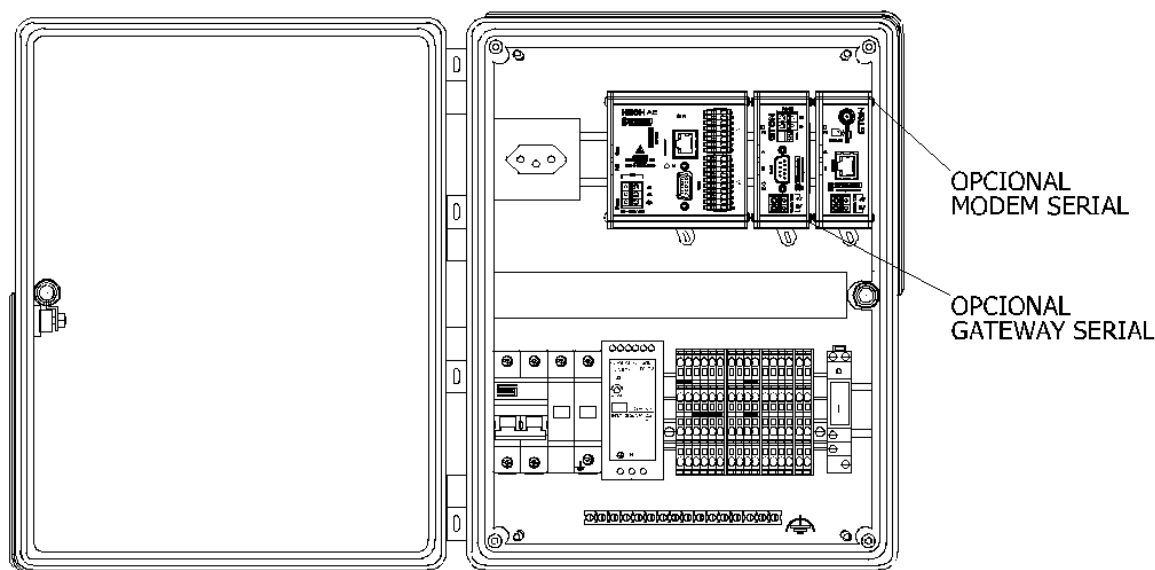
Figura 2 - ACOS225 BM LT, vista frontal, porta aberta
