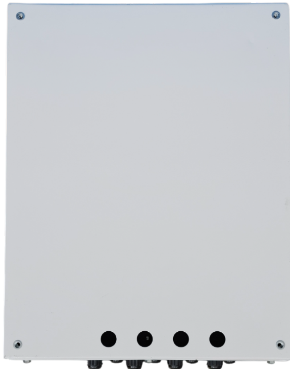
Figura 2 - ACOS500 BM STD com Gateway Modbus, vista traseira para conexão com o painel do inversor de frequência e entrada de cabos
