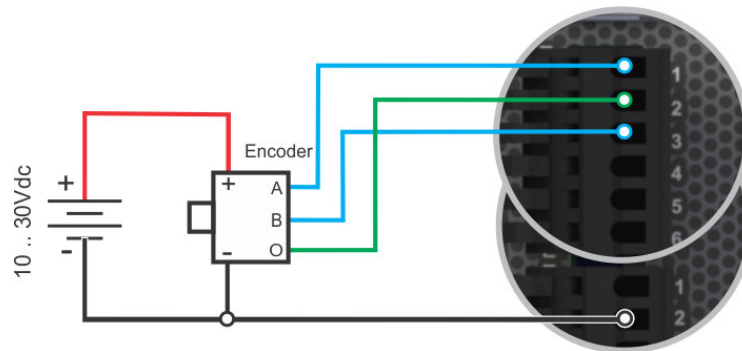
Conexões para utilização do encoder T0, com sinal de sincronismo [O].
