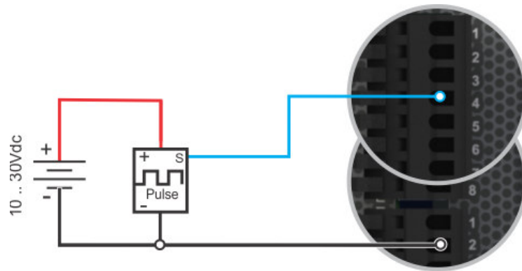
Conexões para utilização da entrada digital I3 como contador rápido T1.
